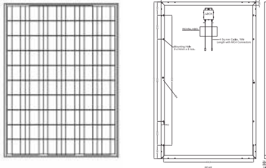
MODULE DIMENSION
