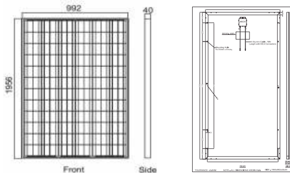
MODULE DIMENSION
