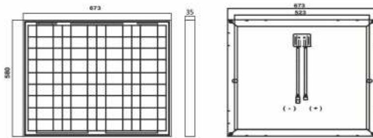
MODULE DIMENSION
